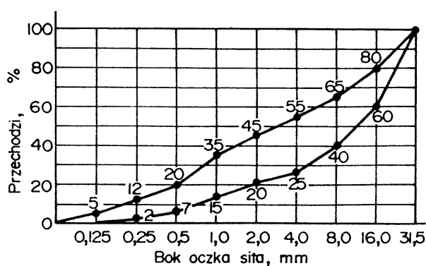
Rysunek 1. Graniczne krzywe uziarnienia do betonu od 0 do 31,5 mm.
